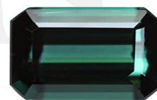
TOURMALINE 碧玺
